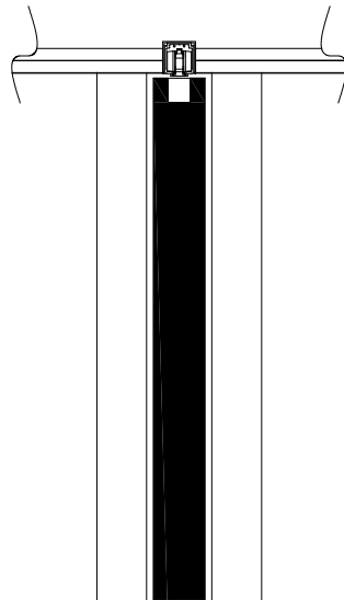
Konstruktionsskinne 36 mm
