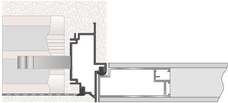
Montering af Dørramme i sten og betonavæg
