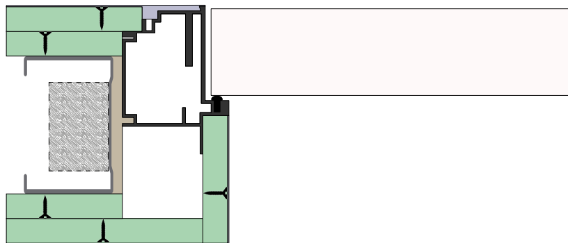
Montering af dørkarm i gipspladevæg
