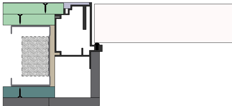
Montering af dørkarm ved panel eller flisevæg
