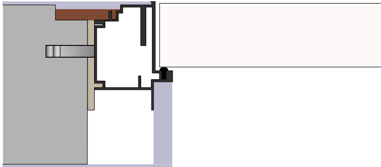
Montering af dørkarm i sten og betonvæg
