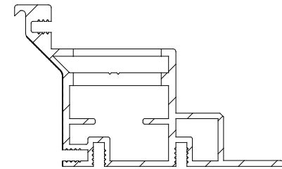
Frameless Door Standard Indadgående profil
